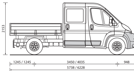
Valník Dvoubakina
